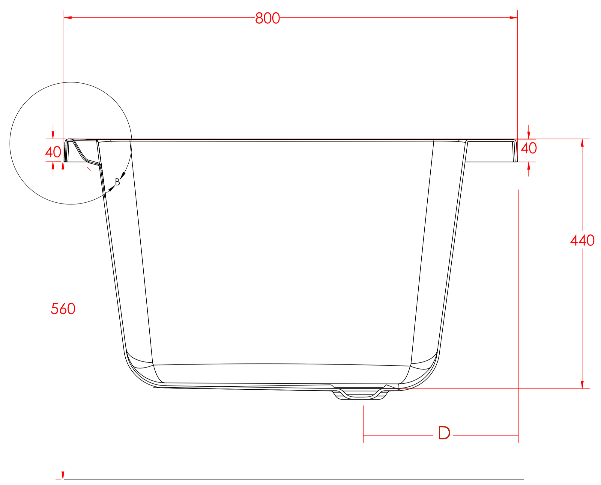
SECTION A-A SCALE 1 : 4
